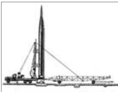
Технологические средства установки Р-5 на пусковой стол
