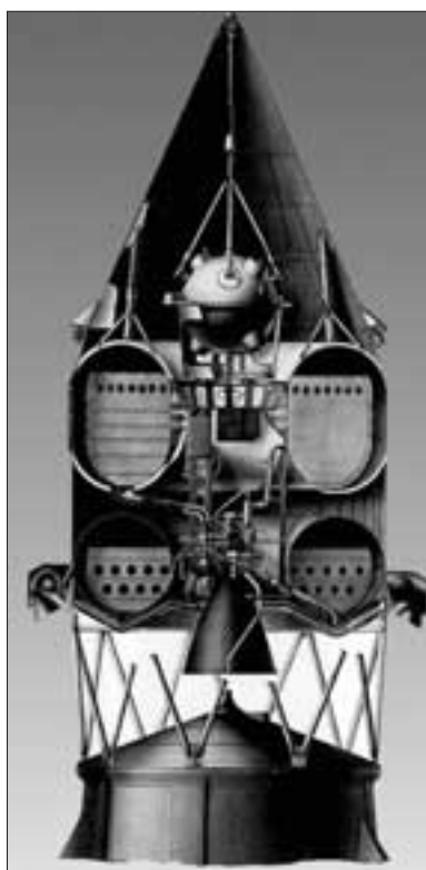
Блок «Е»
