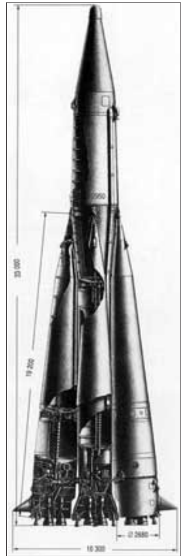
Ракета Р-7
