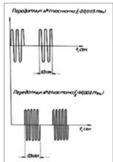
Форма радиосигнала первого искусственного спутника Земли
